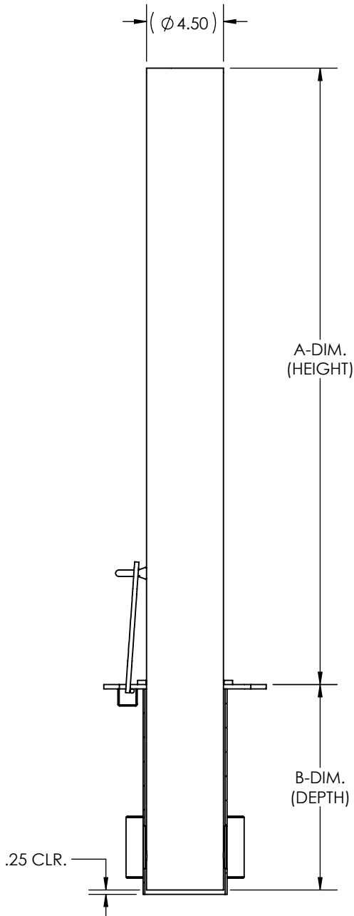
SECTION A-A
